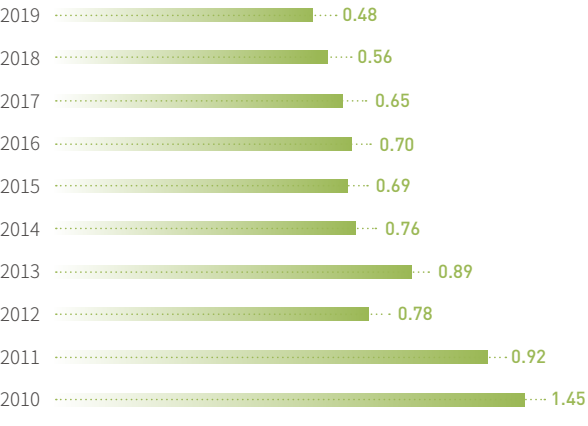
2010-2019 年吨水泥熟料氮氧化物排放量 单位：千克 / 吨
